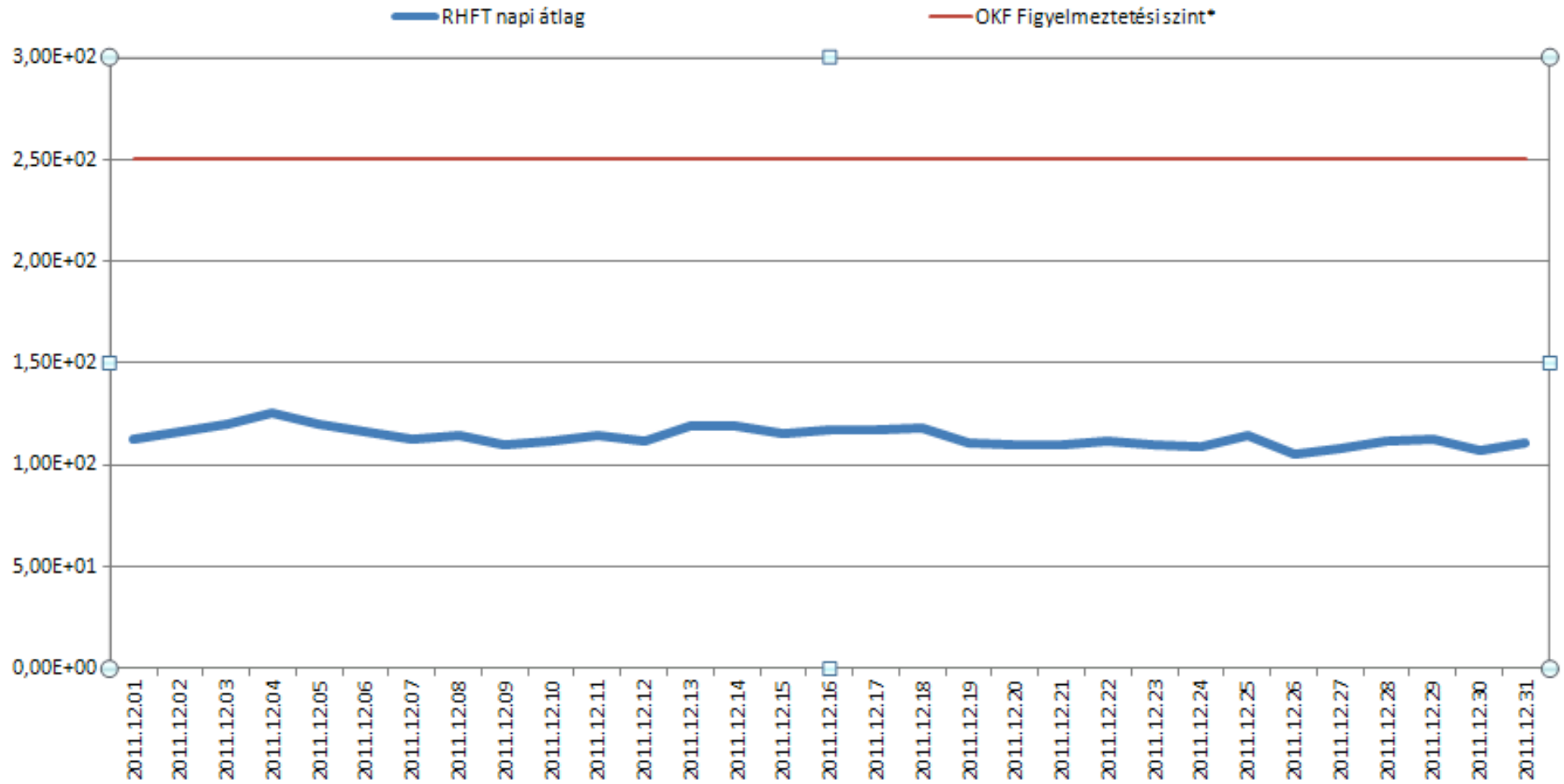
A püspökszilágyi RHFT területén mért dózisteljesítmények napi átlagai 2011 december (nSv/h)
